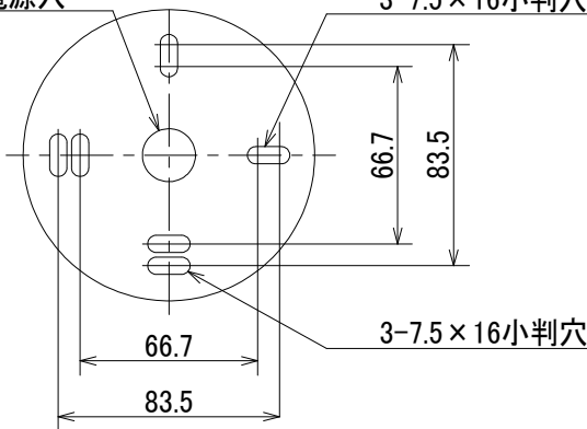
取付寸法図
