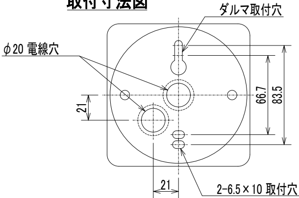
取付寸法図
