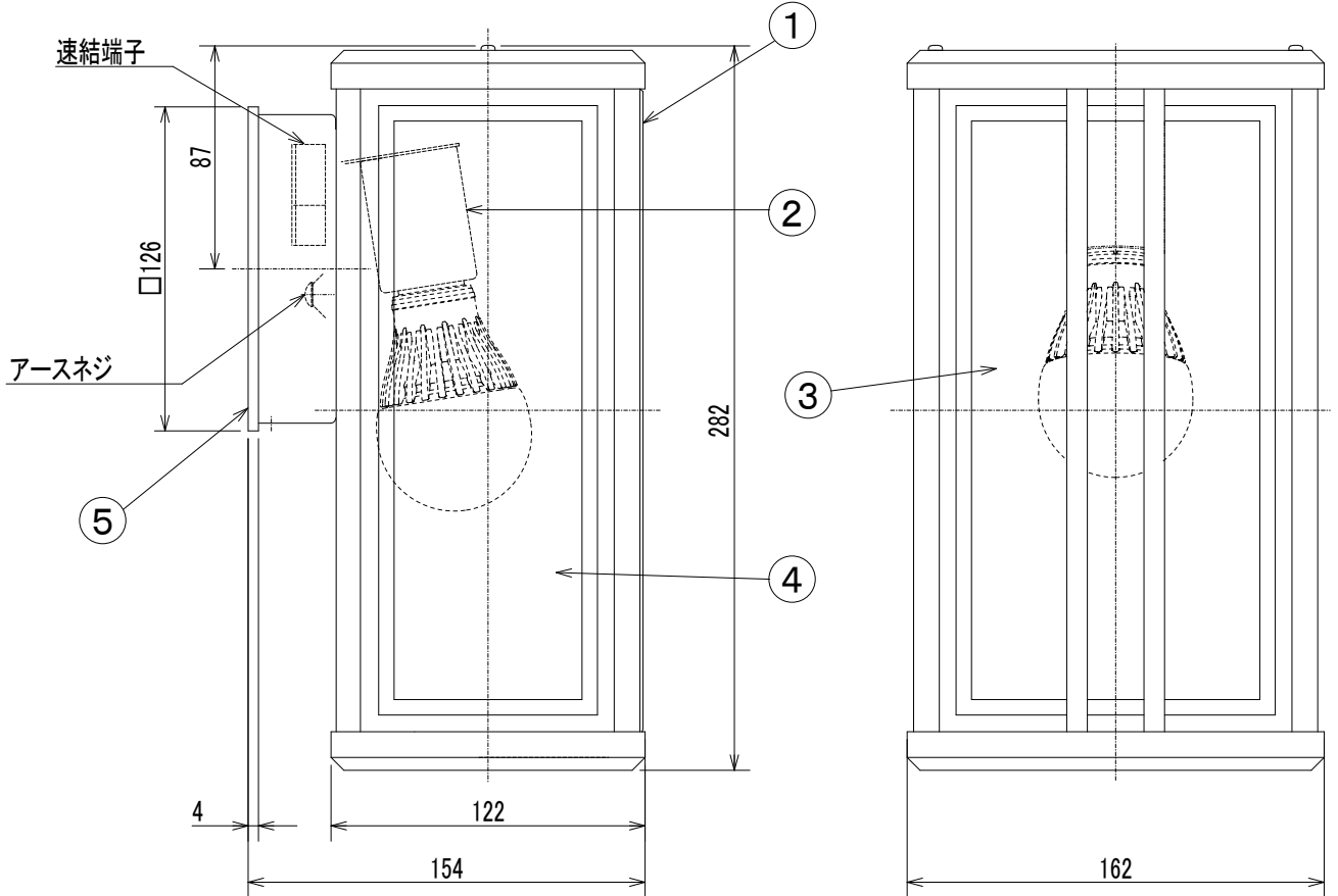
取付寸法図
