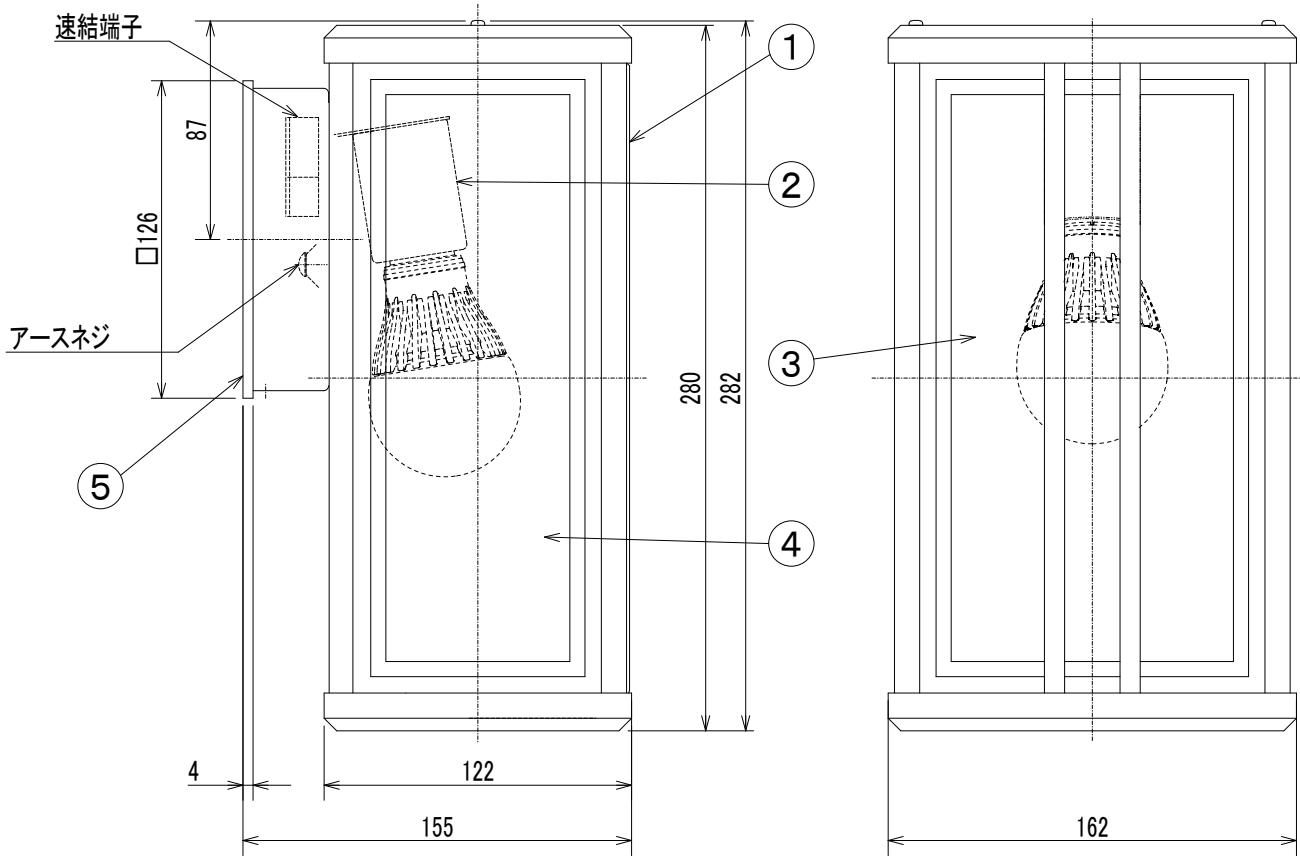
取付寸法図
