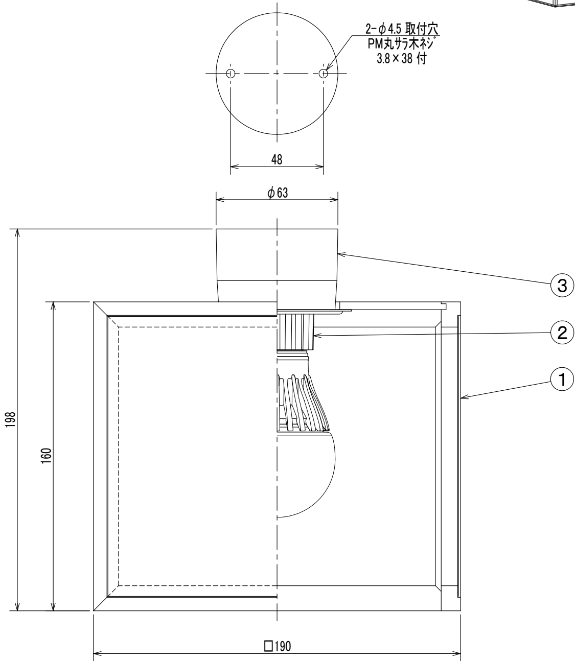
丸形引掛シーリング式
