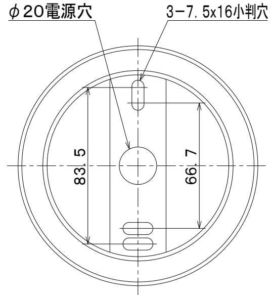
取付寸法図
