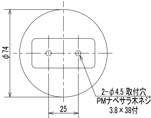
引掛シーリング取付寸法図
