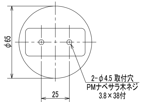
引掛シーリング取付寸法図
