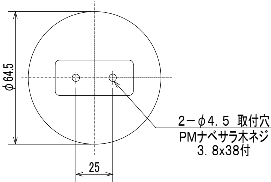
引掛シーリング取付寸法図
