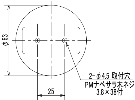
引掛シーリング取付寸法図
