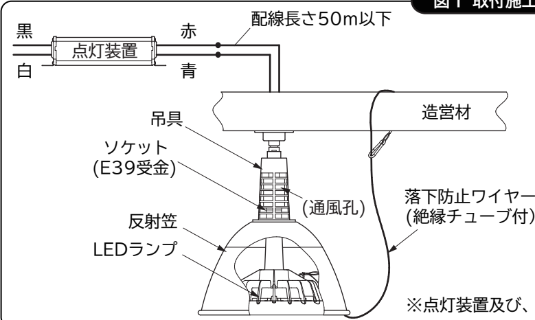
図1 取付施工例
