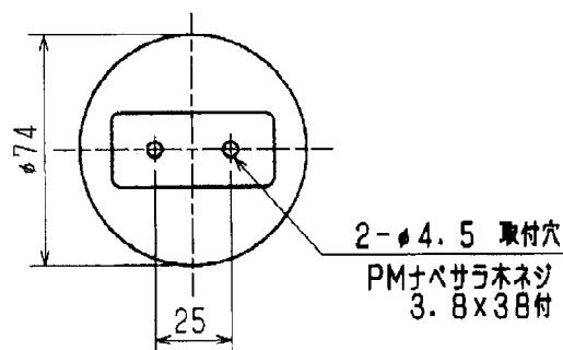
引掛シーリング取付寸法図
