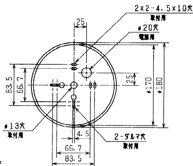
取付寸法図
