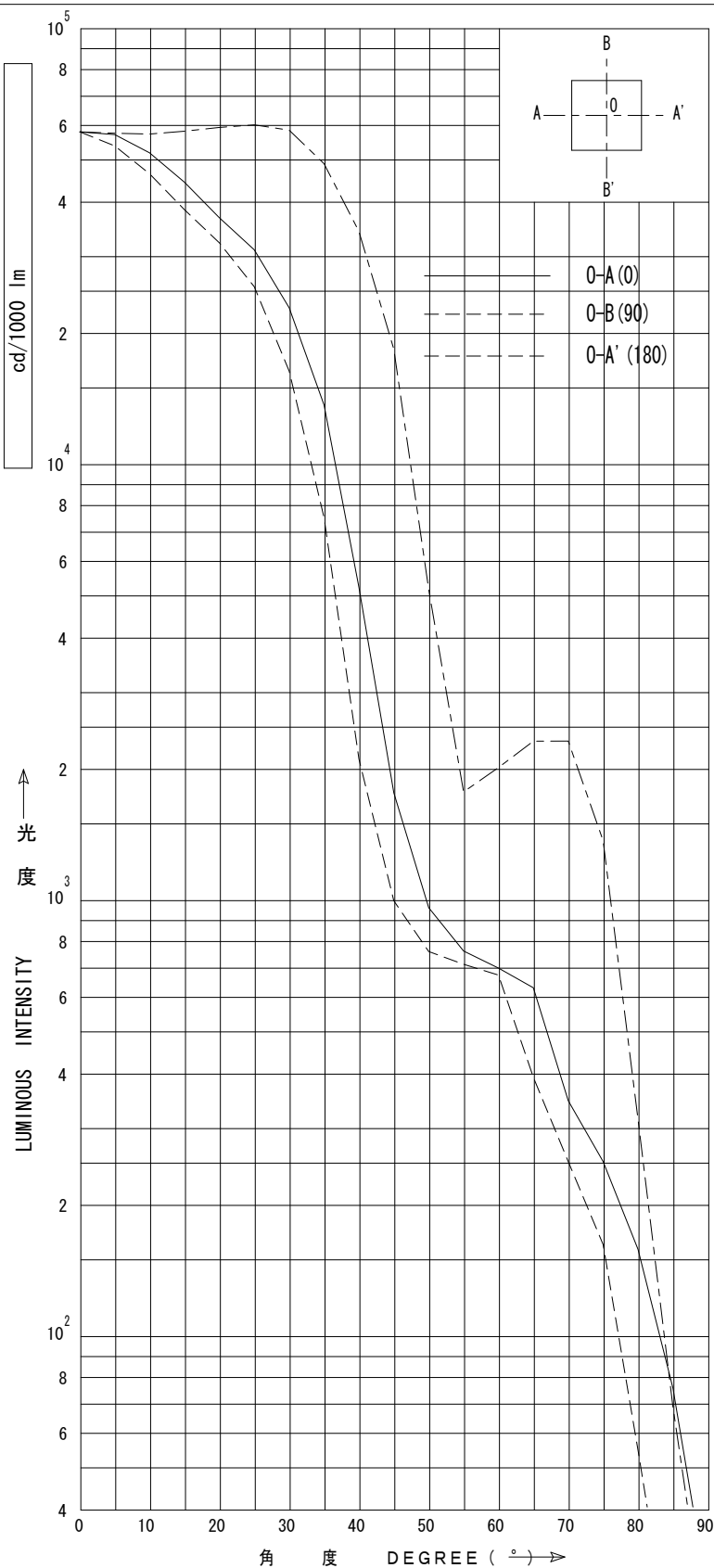
器具形式図 LUMINAIRE FORM
