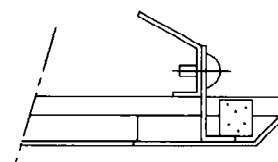
A 部詳細
