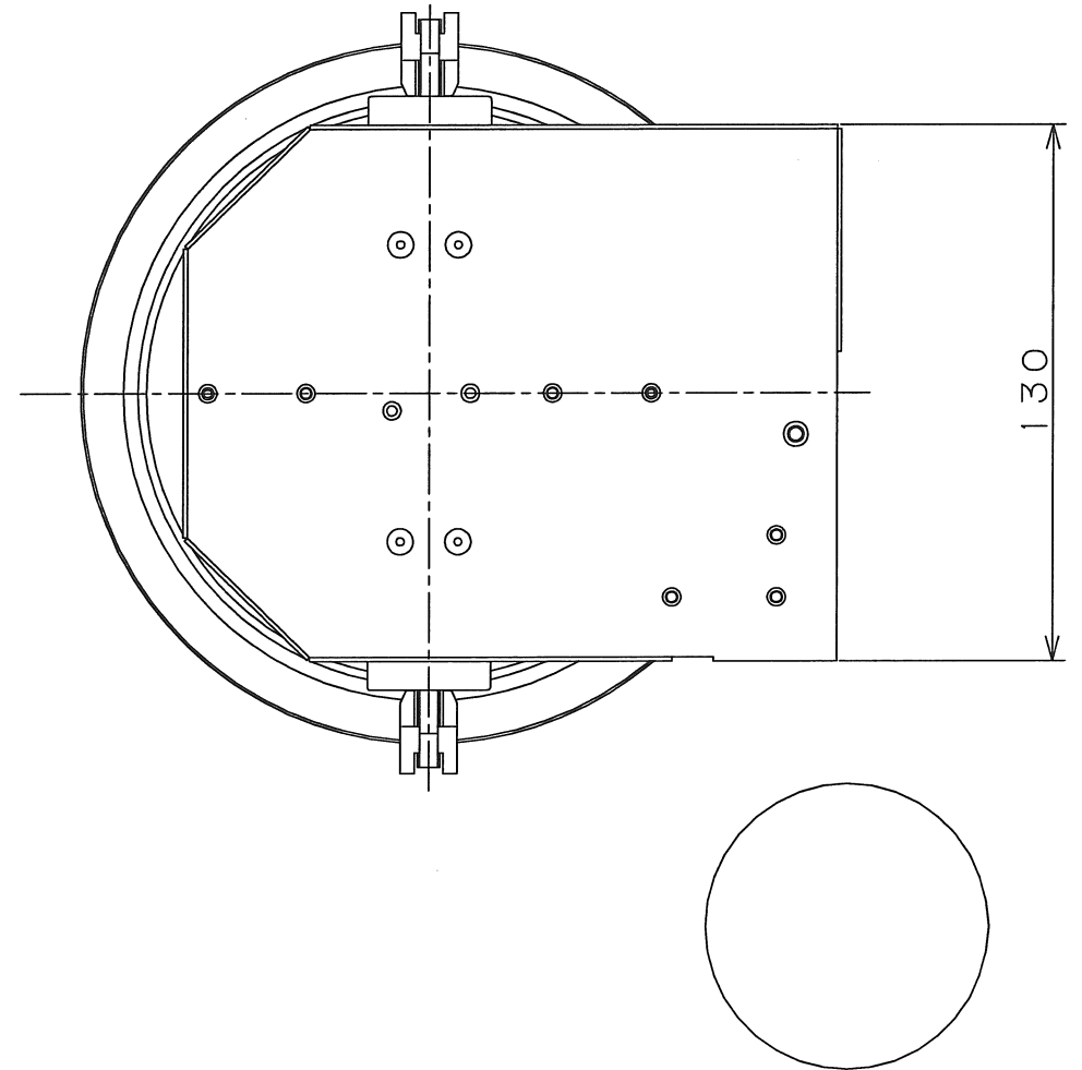
天井切込み寸法 \phi 150
