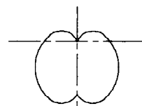
配光パターン
