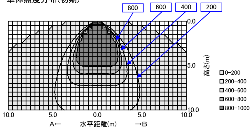
单体照度分布(初期)
