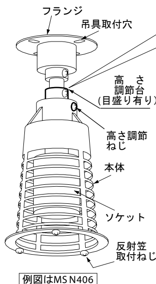
吊具の高さ調節 (図1)
