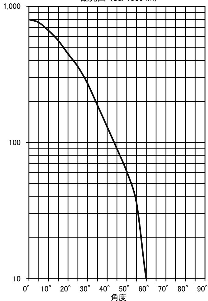
光度 (cd) 配光図 (cd/1000 lm)
