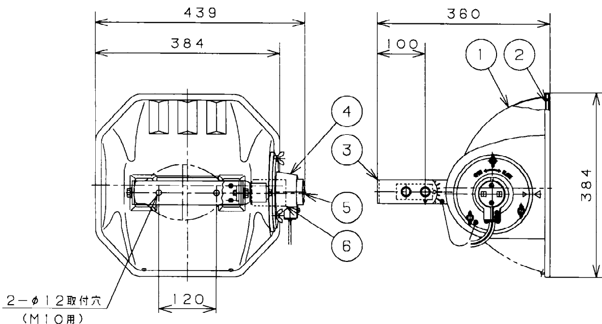
器具の取付方向と可動範囲
