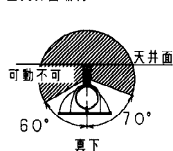
器具の取付方向と可動範囲
