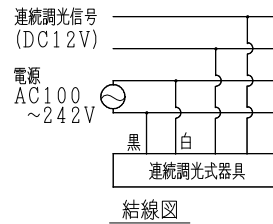
結線図
