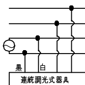
結線図
