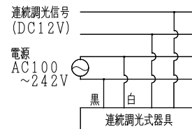
結線図
