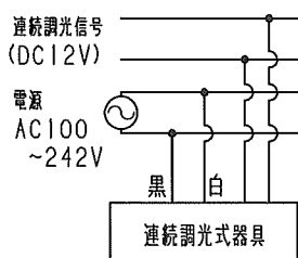
結線図
