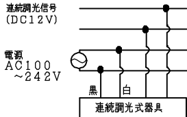
結線図
