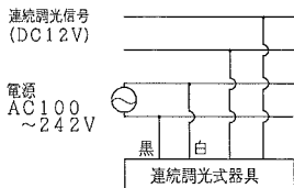
結線図
