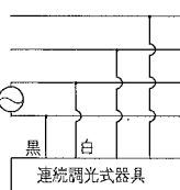
結線図
