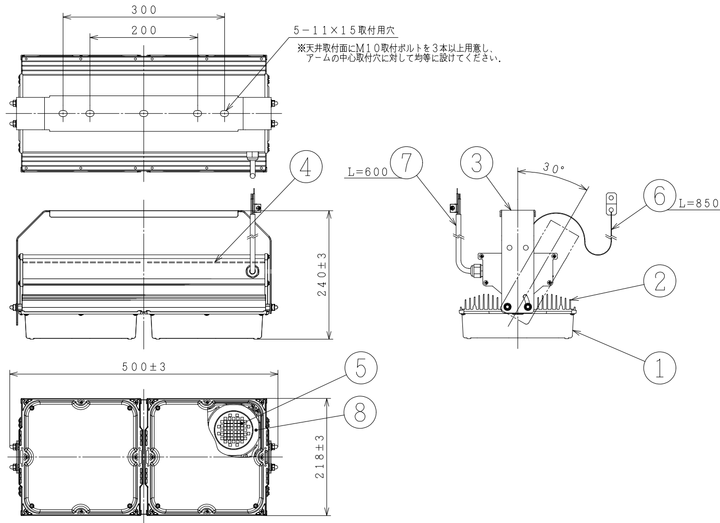
公共施設形 LSR2W-400
