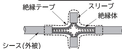
電線接続方法の例(図4)
