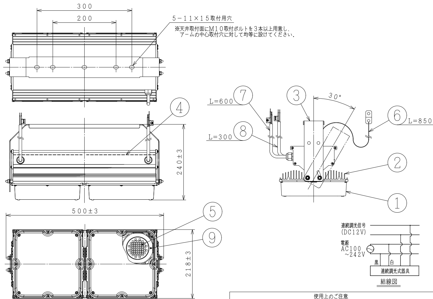
連続調光形 (OFF機能付) 調光範囲: 100～約20%
