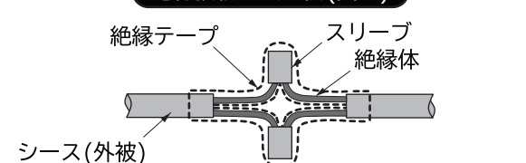
電線接続方法の例(図4)
