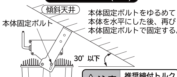
傾斜天井への取付(図3)
