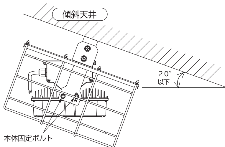
傾斜天井への取付 (図1)
