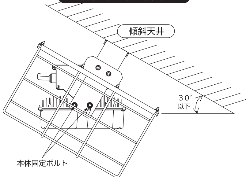
傾斜天井への取付 (図1)
