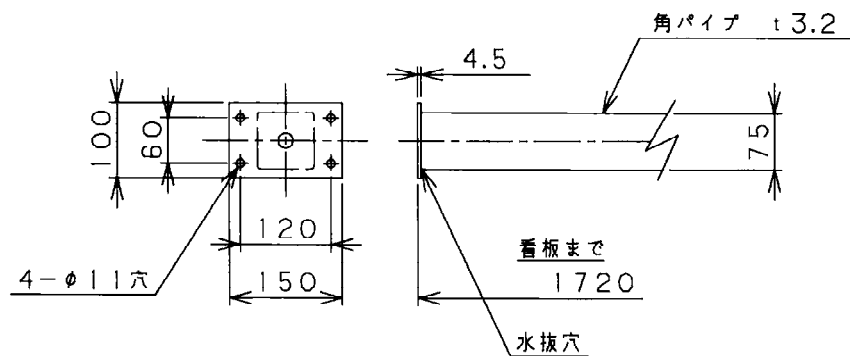
器具取付用アーム 参考図
