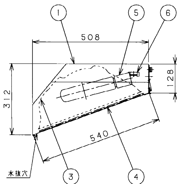
器具取付用アーム 参考図
