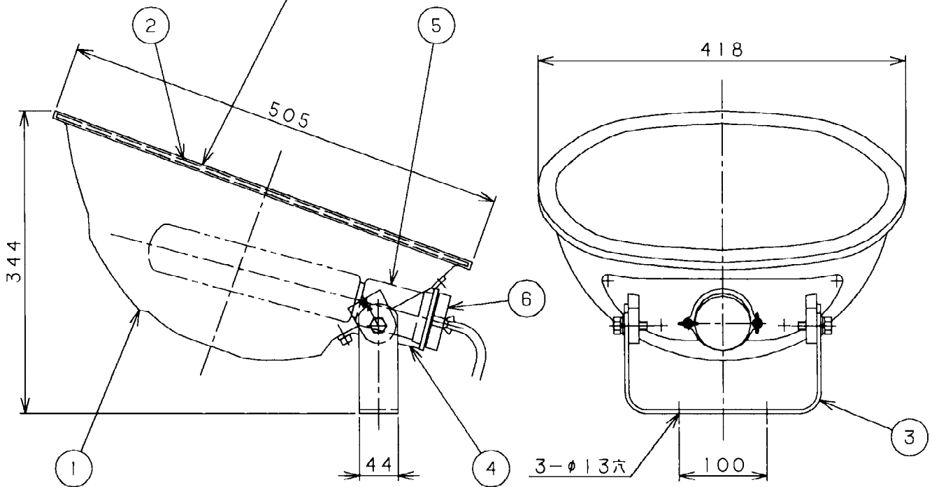
器具取付用アーム 参考図
