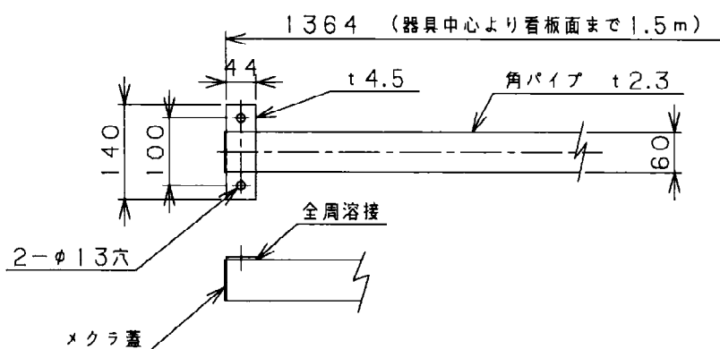
器具取付用アーム 参考図
