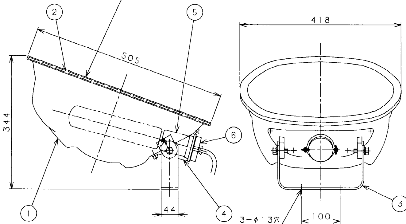
器具取付用アーム 参考図
