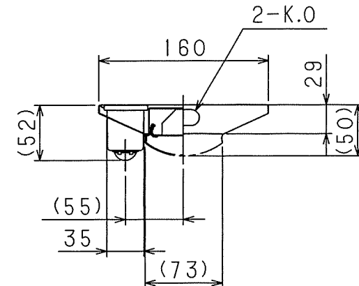
側面詳細図 (S=1:5)
