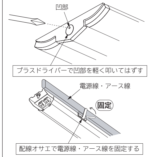
電源端子台の接続と解除 (図3)
