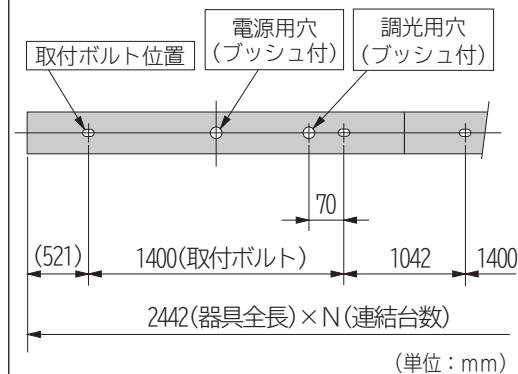
器具内で送り配線する場合 (図2)
