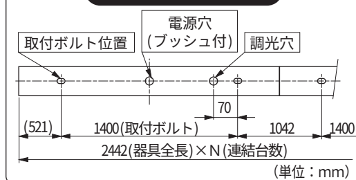
器具内で送り配線する場合 (図2)
