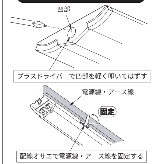
電源端子台の接続と解除 (図3)
