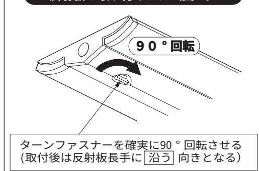
反射板の取り付けかた (図5)
