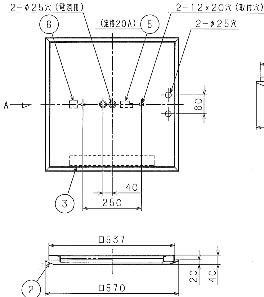
A 矢視
