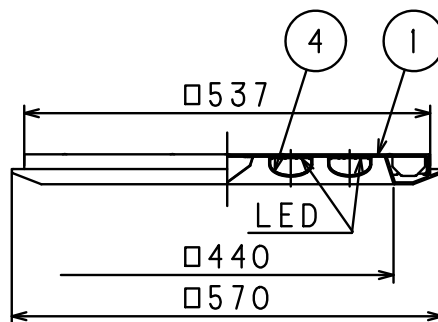
A 矢視
