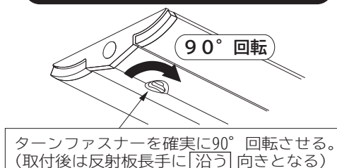
反射板の取り付けかた (図5)
