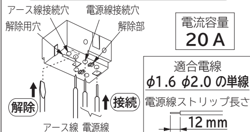
調光端子台の接続と解除 (図4)
