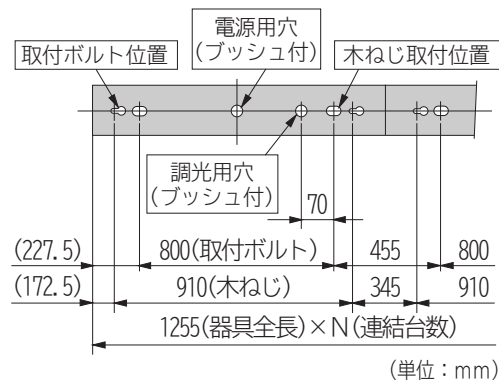
器具内で送り配線する場合 (図2)
