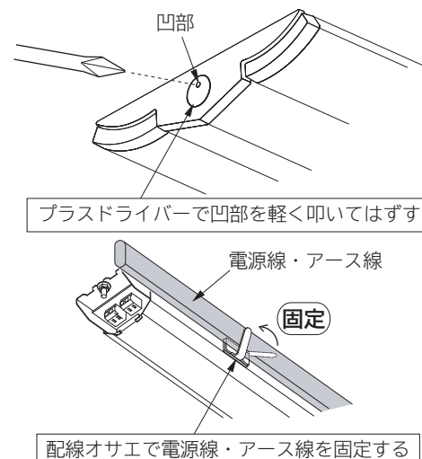
電源端子台の接続と解除 (図3)
