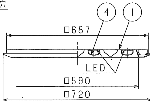
A 矢視
