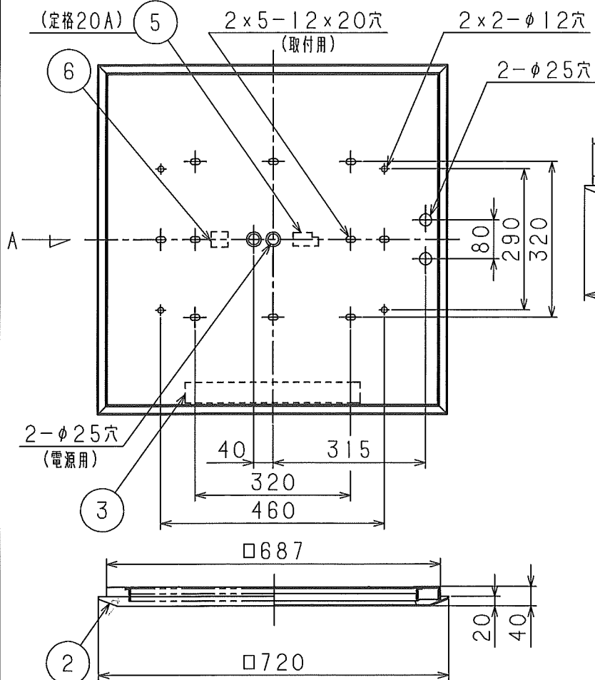
A 矢視
