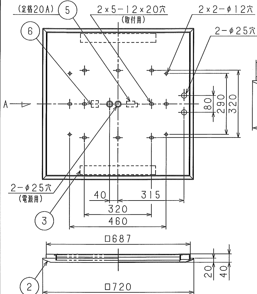
A 矢視
