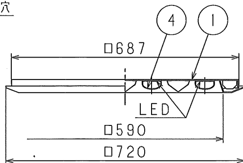
A 矢視
