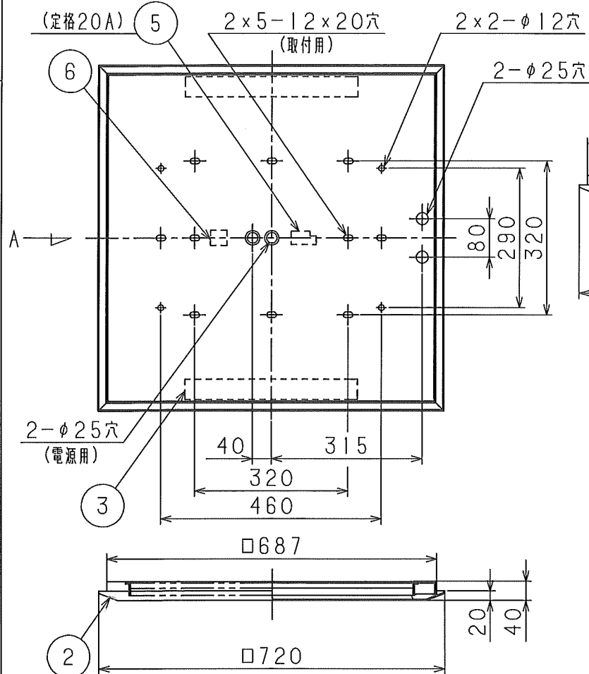
A 矢視
