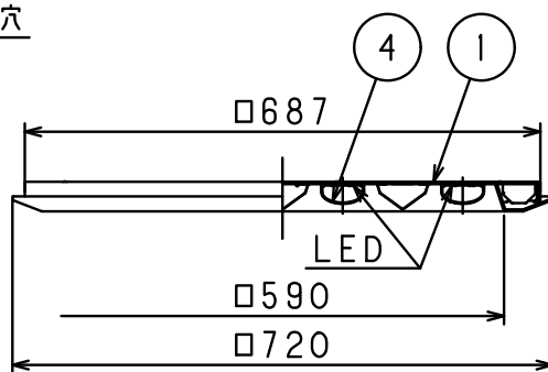
A 矢視
