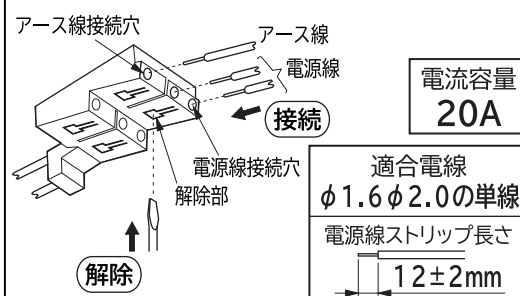
調光端子台の接続と解除(図3)
