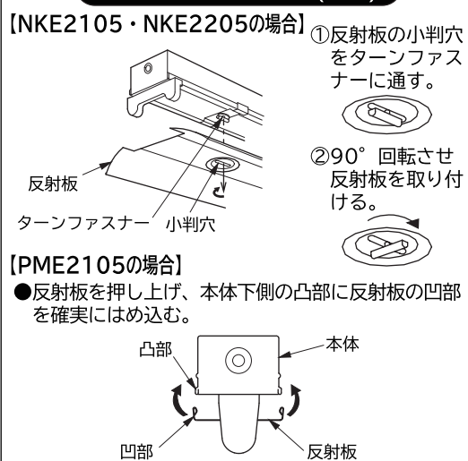
反射板の取り付けかた(図3)
